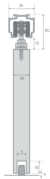
Vista Lateral
